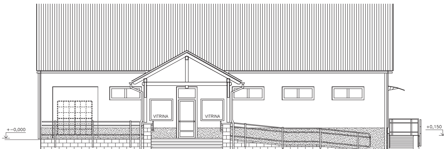
POHLED BOČNÍ - VÝCHODNÍ
