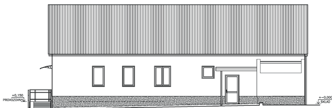
POHLED DVORNÍ - SEVERNÍ
